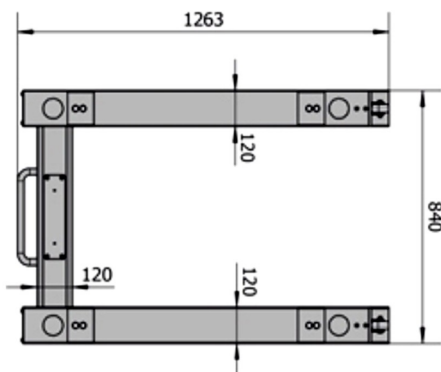
PALETTENWAAGE IHG-PLW
