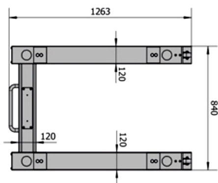
PALETTENWAAGE IHG-PLW
